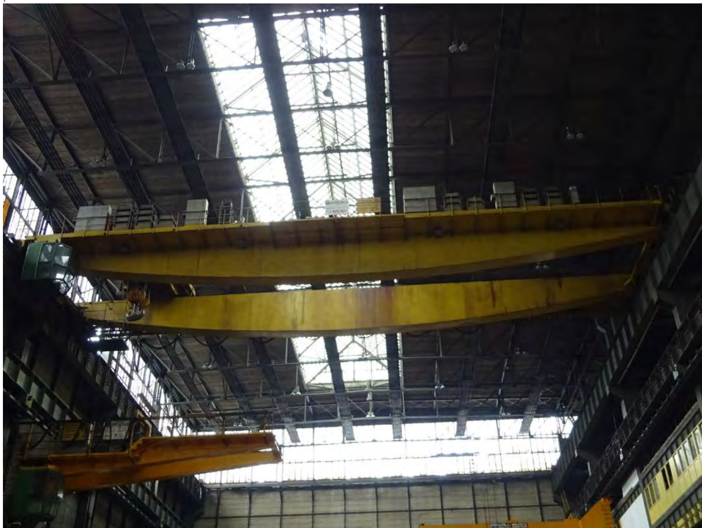
... 741. .... • DVOGREDNA MOSNA DIZALICA, .... DMD 125/10 Mp / 33m..... ..88.
