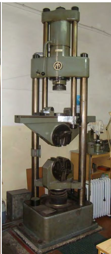
... 61. .... • STROJ za vlačno ispitivanje materijala, ..... UPD 600.....
